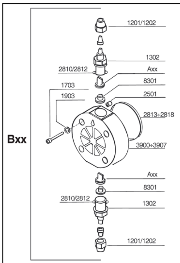
ГОЛОВКА 3 ПП, ПВХ, Н/СТ, ТЕФЛОНА
