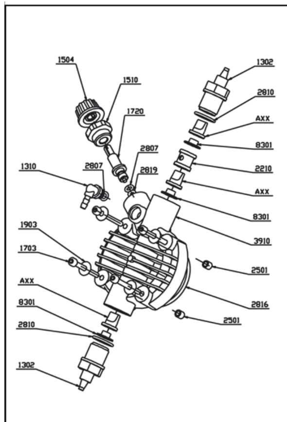
СТАНДАРТНА ГОЛОВКА З РУЧНИМ КЛАПАНОМ СТРАВЛЮВАННЯ ПОВІТРЯ
