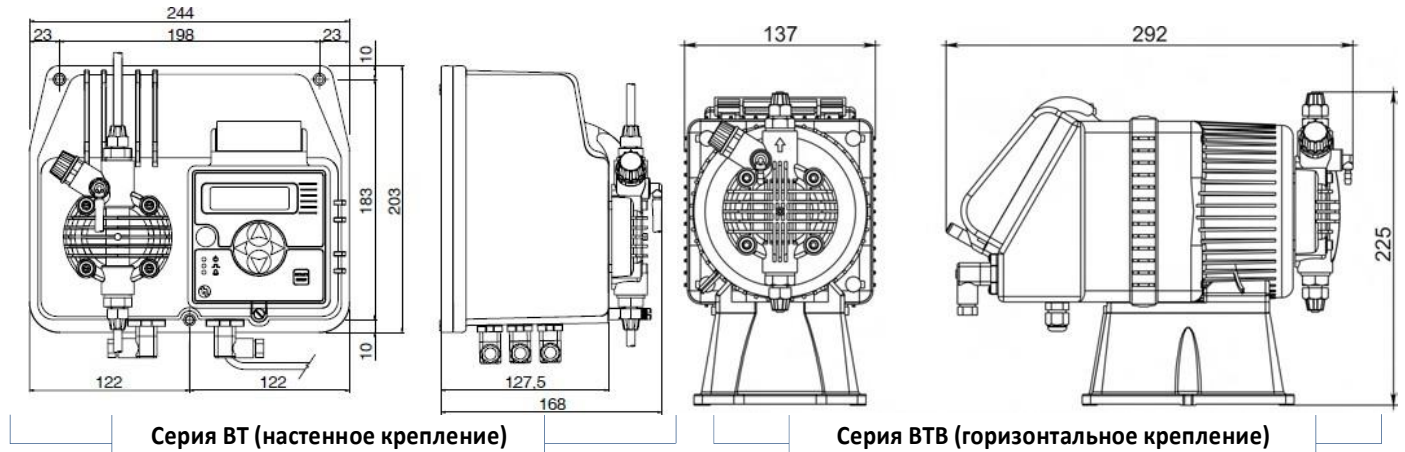
ЗАГАЛЬНІ РОЗМІРИ (Рис. 1)
